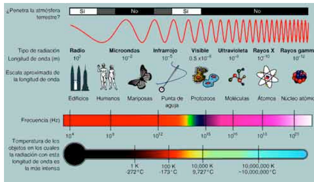
Figura 1. El espectro electromagnético como función de la frecuencia y la longitud de onda.
