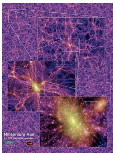
Figura 5. La distribución de la materia a grandes escalas. Cada punto luminoso es un fuerte candidato a crear una galaxia.
